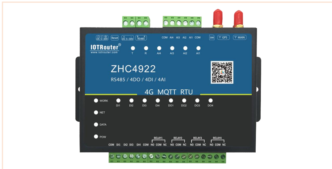
图 1 外观说明
